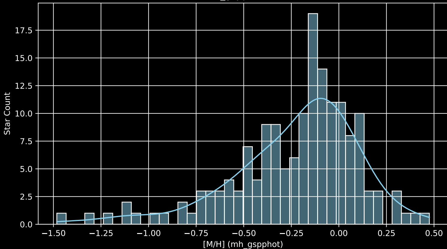
APOGEE DR17 Field: [283-22-O_TESS [M/H] (mh_gspphot) (n= 162)
