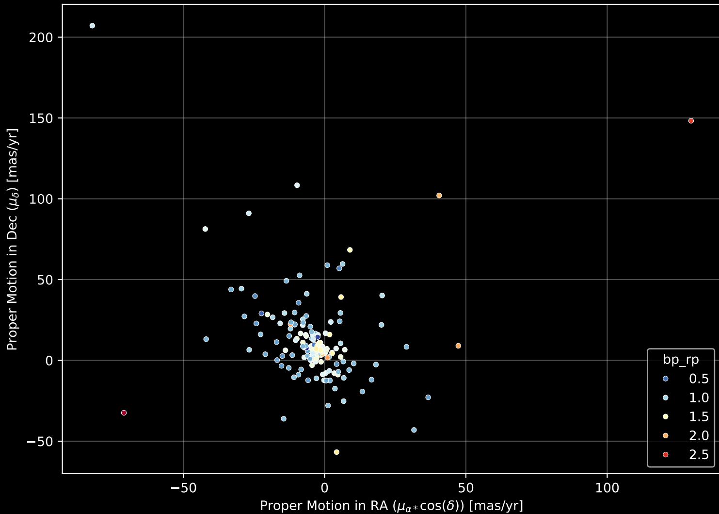
APOGEE DR17 Field: [283-22-O_TESS] Proper Motion Diagram (n= 163)
