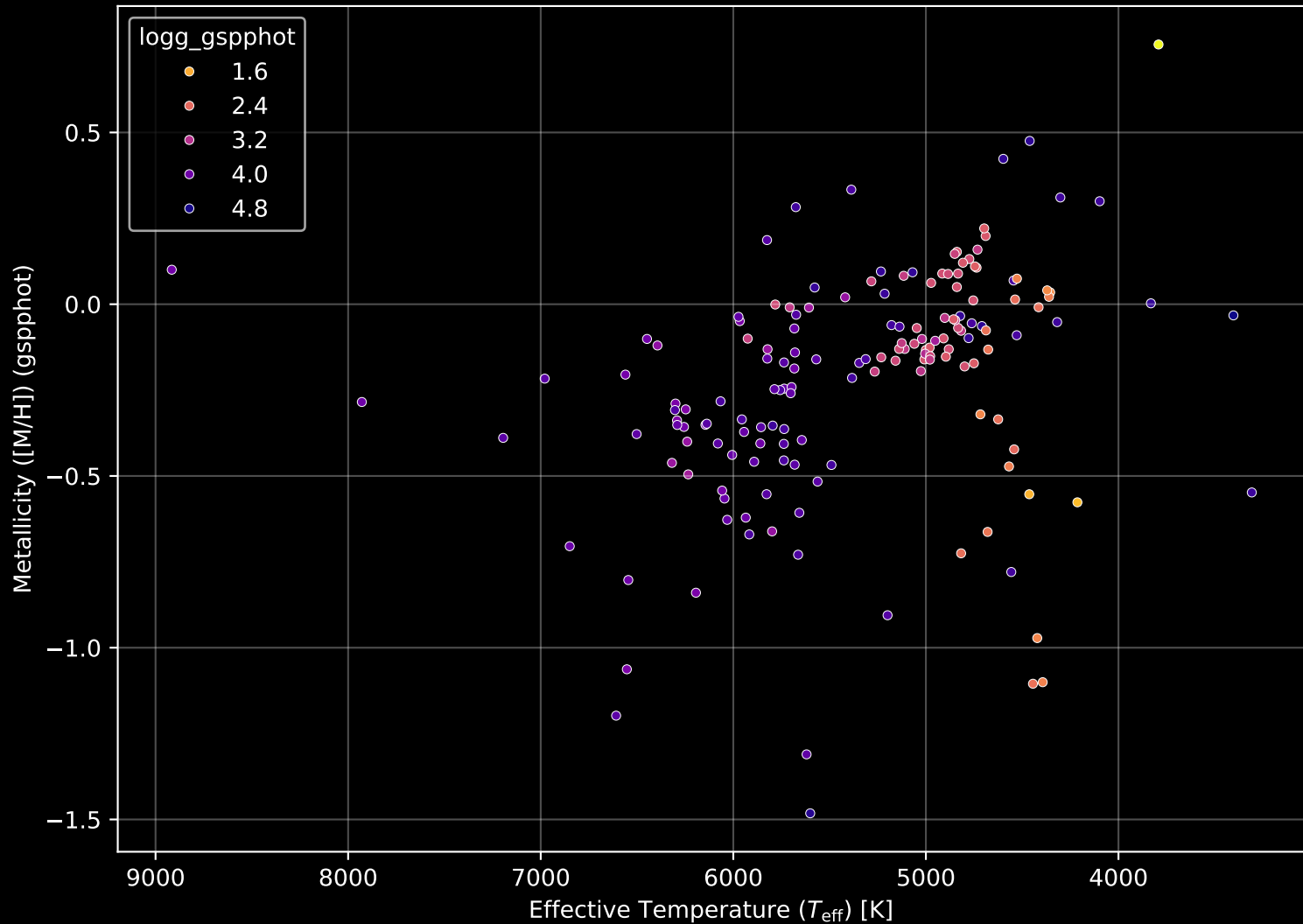
APOGEE DR17 Field: [283-22-O_TESS] Stellar Population Parameters (n= 163)
