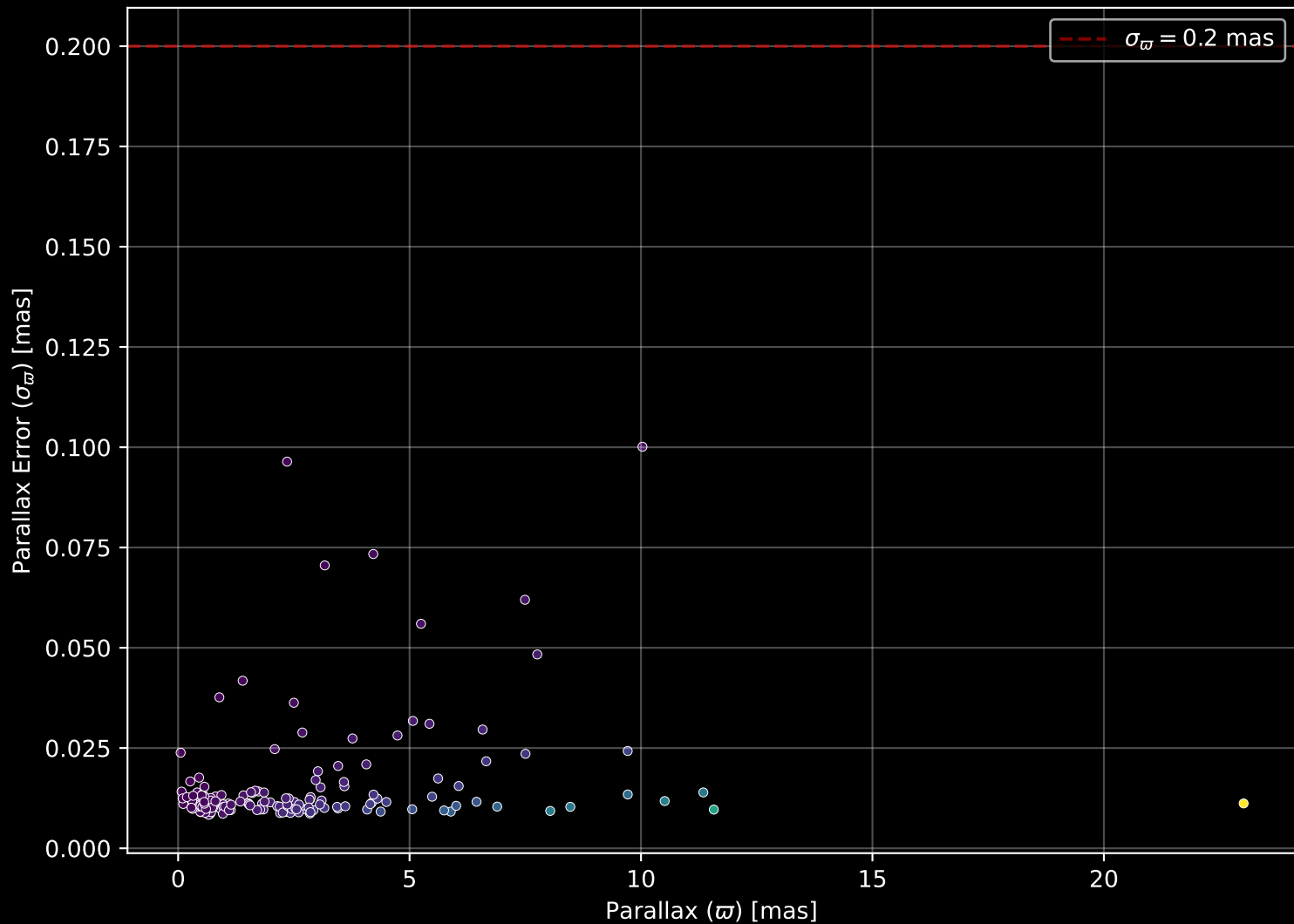
APOGEE DR17 Field: [283-22-O_TESS] Parallax Quality (n= 163)
