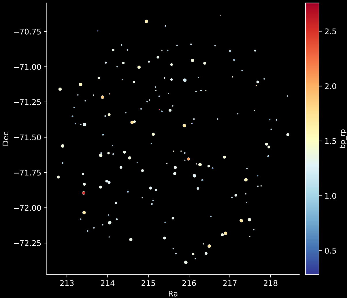
APOGEE DR17 Field: [283-22-O_TESS] Stars: 163
